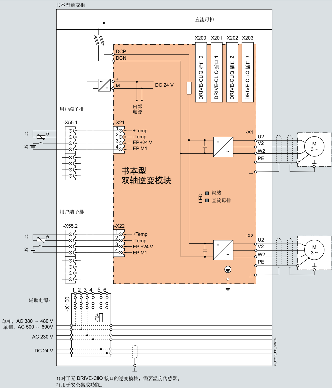
连接示例：装柜的书本型双轴逆变模块
