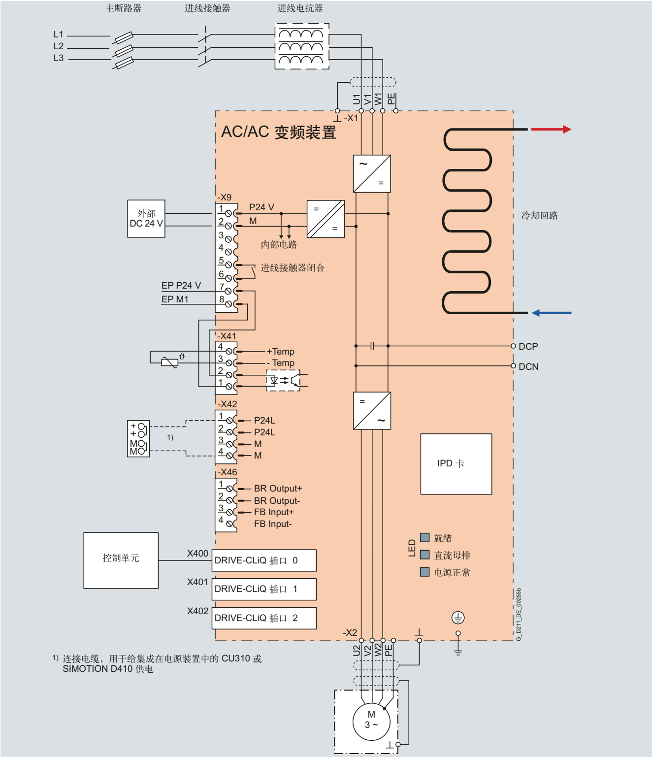
连接示例：水冷式 AC/AC 变频调速装置
