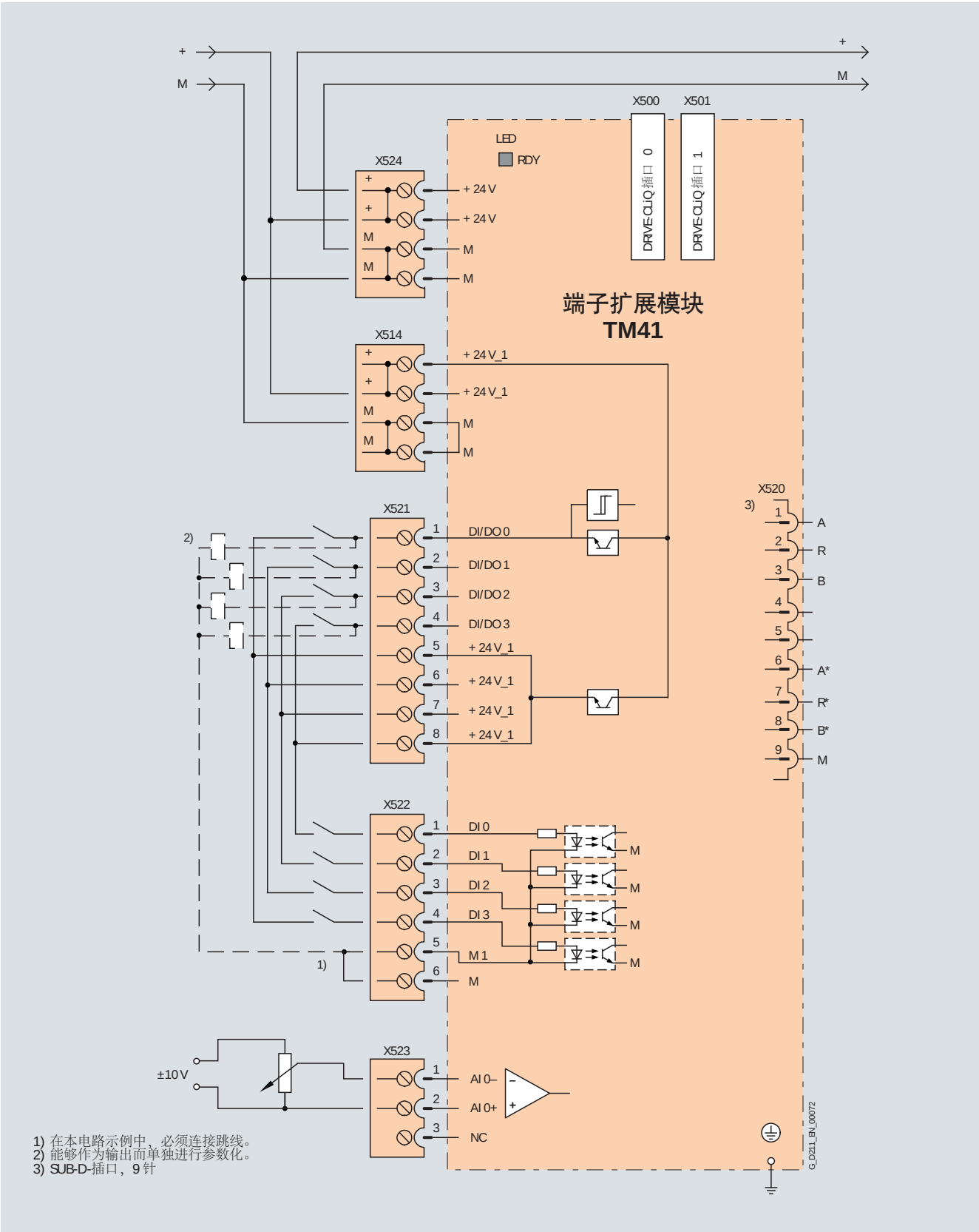
连接示例：端子扩展模块 TM41
