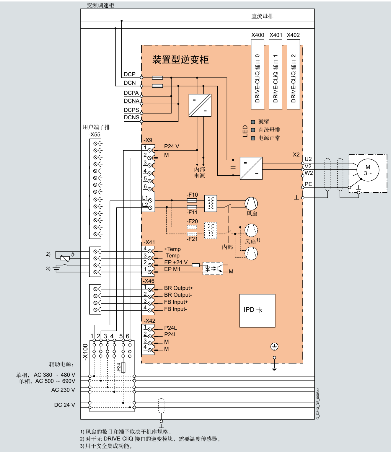
连接示例：装置型逆变柜
