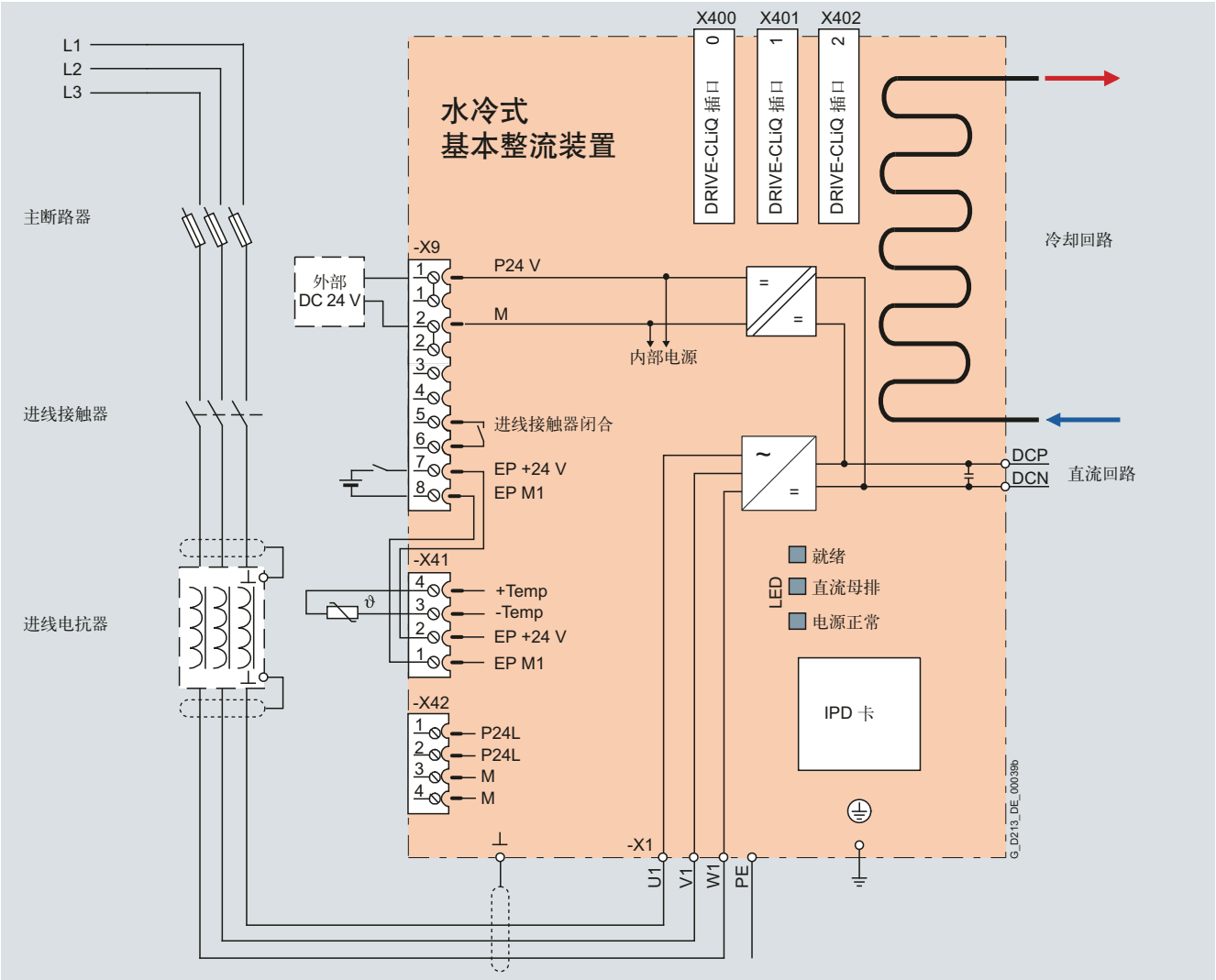
连接示例：基本整流装置
