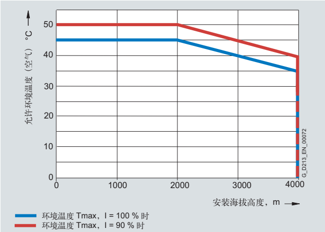
不同环境温度与安装海拔高度下的降容
