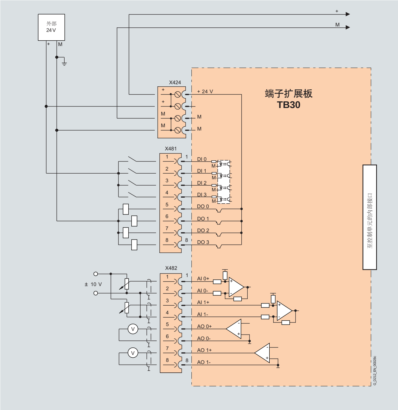
连接示例：端子扩展板 TB30
