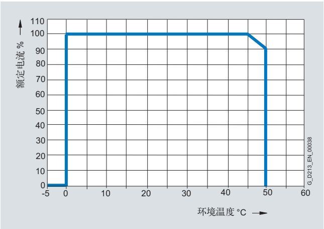
不同环境温度下电流降容
