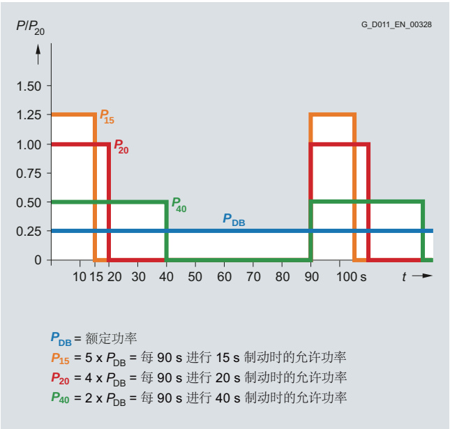
制动单元和制动电阻的负荷曲线
