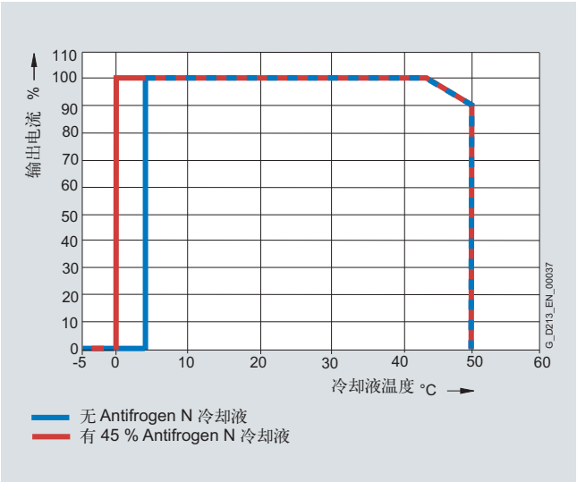
不同冷却液温度下电流降容
