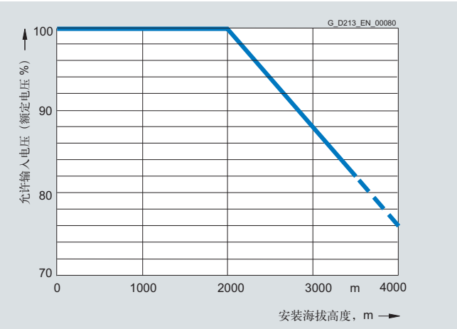
不同安装海拔高度下的电压降容
